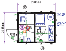
Módulo sanitario de 10'
