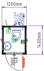
Cabina sanitaria de 5'
