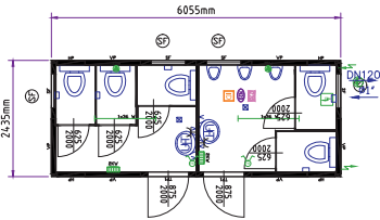
Cabina sanitaria de 20' hombres / mujeres
