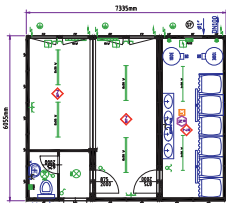
Módulo de oficina y sanitarios (conjunto triple)
