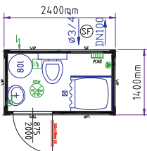
Cabina sanitaria/duchas de 8'
