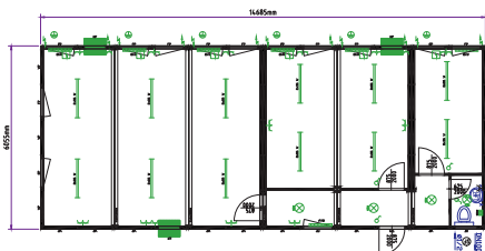
Módulo de oficina y sanitarios (conjunto séxtuple)
