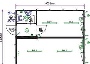
Módulo de oficina y sanitarios (conjunto doble)
